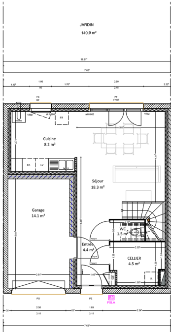
PLAN RDC
